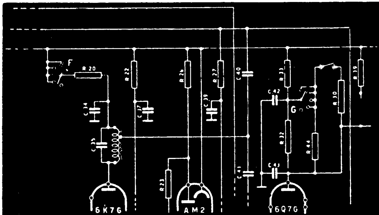
LA VOCE DEL PADRONE — Al telaio del mod. 835 e 1835 è stata appor- tata la seguente variante circuitale: Connessioni delle sezioni F e G, del commutatore modificate come da disegno allegato.
